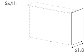
TBF7 L1,8 P61,8 H107,2 TBF6 L1,8 P61,8 H107,2
