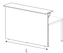
TBF12 L120 P40 H110,4 TBF14 L140 P40 H110,4 TBF16 L160 P40 H110,4 TBF18 L180 P40 H110,4 TBF20 L200 P40 H110,4
